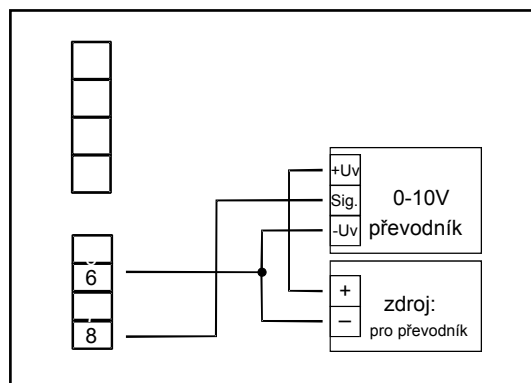
převodník 0-10V (připojení 3-vodičovou technikou)
