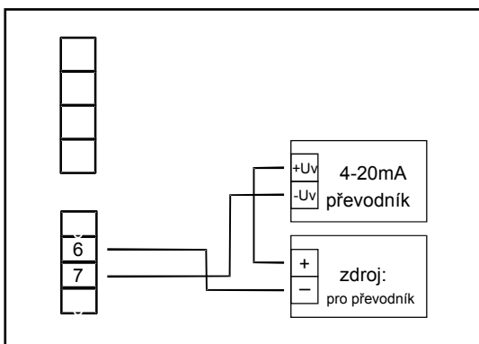
převodník 4-20mA (připojení 2-vodičovou technikou)
