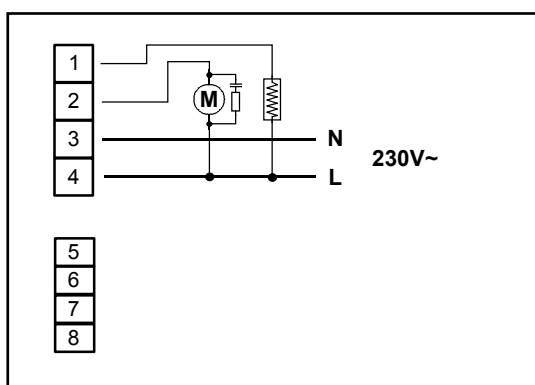
připojení spotřebiče (motor, topení)
